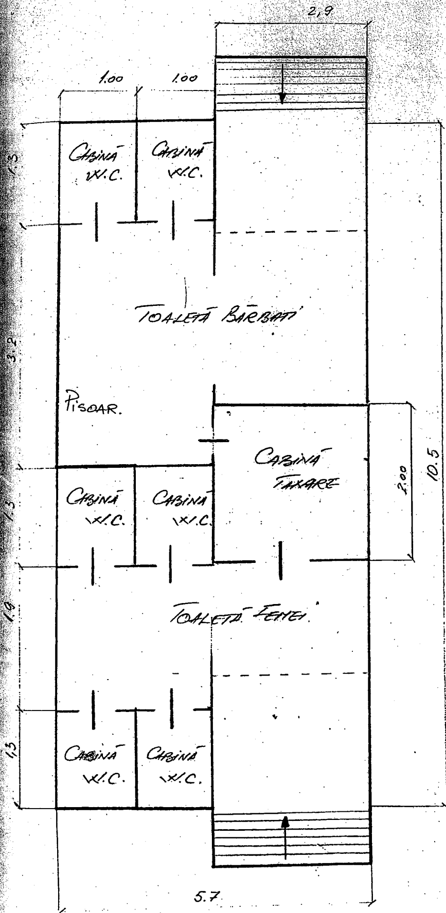
PLAN RELEVU - TOALETĂ PUBLICĂ (PIATA CATEDRALEI)
