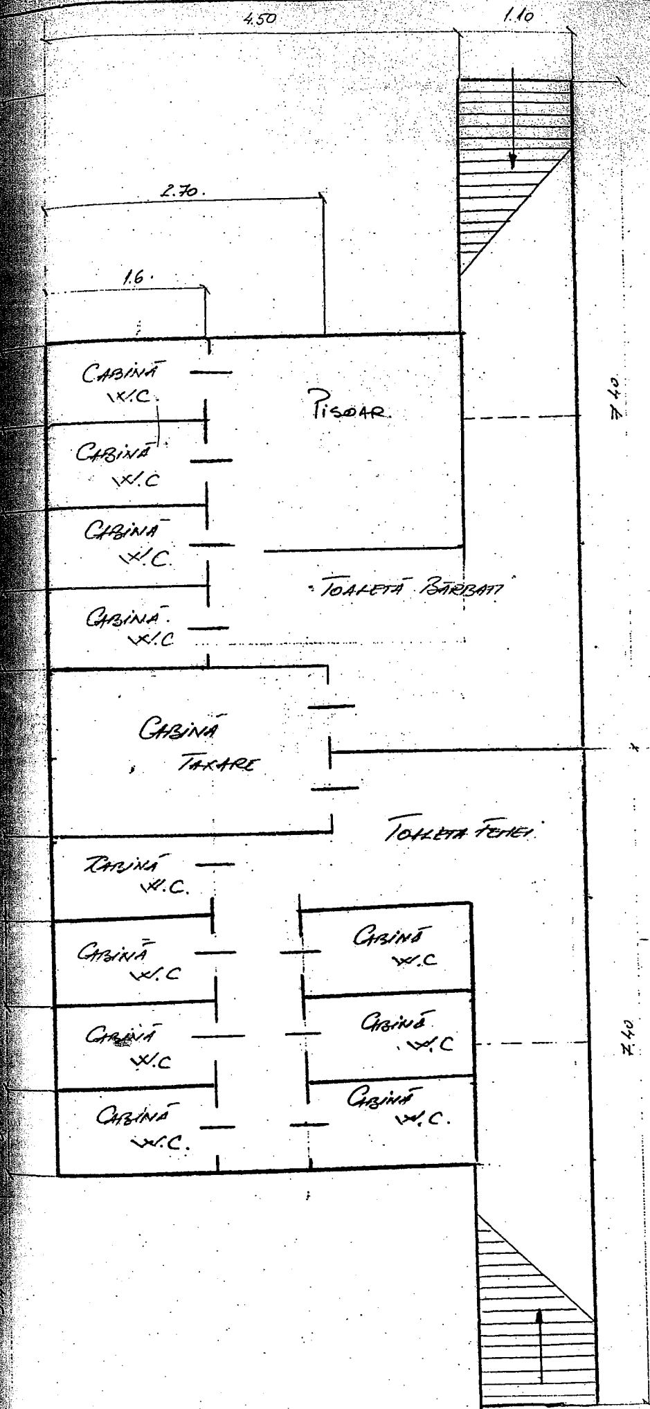
PLAN REZERVEU - TOILETĂ PUBLICĂ (BULEVARD - LIBERU)
