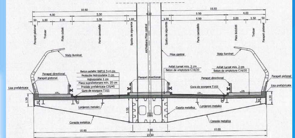
SECTIUNE TRANSVERSALA POD HOBANAT Scara 1:100
