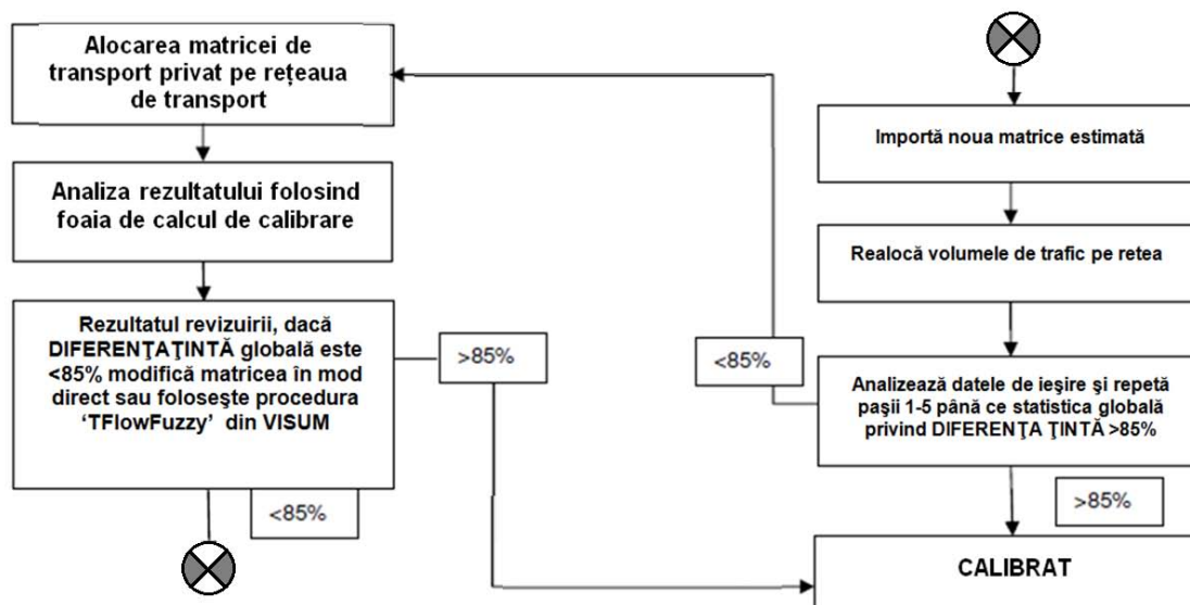
FIGURA 70: PROCESUL DE CALIBRARE A MODELULUI DE TRANSPORT PENTRU MATRICEA DE TRANSPORT PRIVAT
