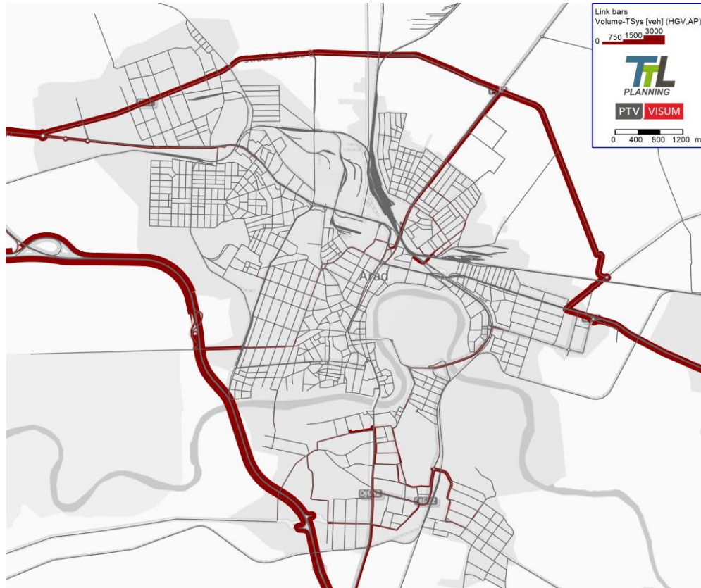
FIGURA 80: MĂRIMEA FLUXURILOR RUTIERE DE TRAFIC - VEHICULE GRELE DE MARFĂ – PROGNOZĂ 2025
