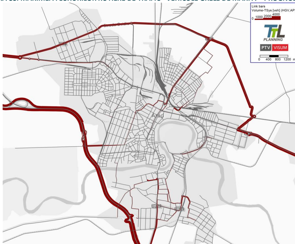
FIGURA 88: MĂRIMEA FLUXURILOR RUTIERE DE TRAFIC - VEHICULE GRELE DE MĂRFĂ – PROGNOZĂ 2035
