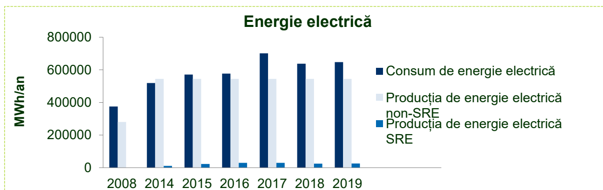
Fig. 17 Producția locală de energie - energie electrică pentru perioada 2014 -2019, față de anul de referință 2008
