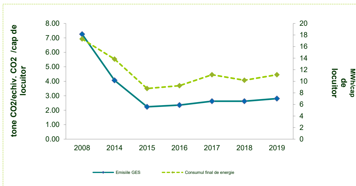
Fig. 13 Emisiile de gaze cu efect de seră (GES) și consumul final de energie pe cap de locuitor pentru perioada 2014 - 2019, față de anul de referință 2008
